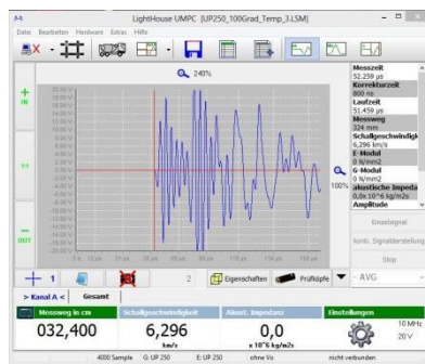
Laufzeitsignal
