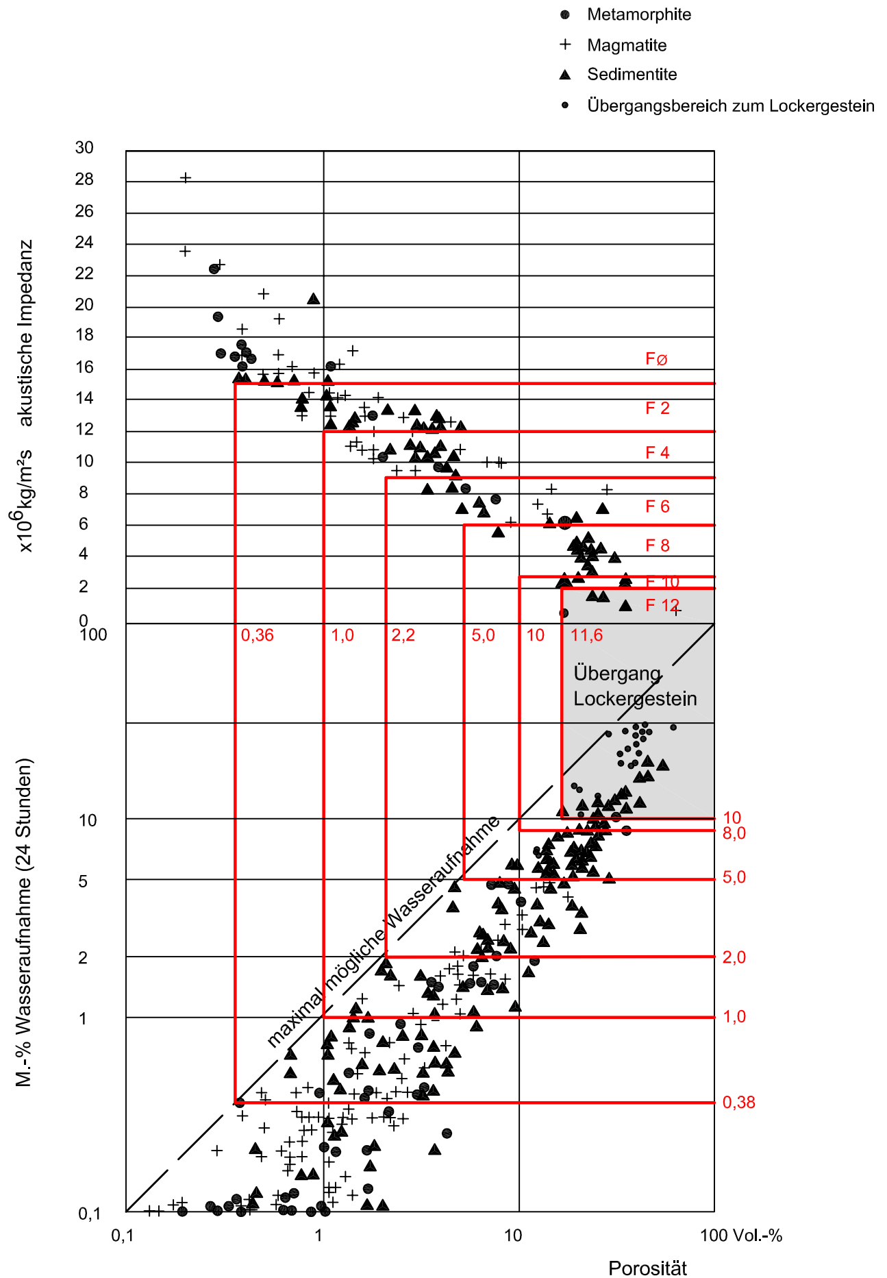
Bild 5: Einteilungsmöglichkeiten der Festgesteine hinsichtlich der akustischen Impedanz ( 10^6 \text{ kg/m}^2 \text{ s} ) und deren Zusammenhänge mit der Porosität (Vol.-%) und Wasseraufnahme (M.-%)
